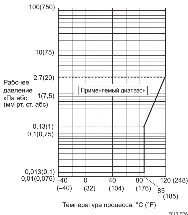
Рисунок 1-1. Рабочее давление и температура процесса [для модели EJX510A]
