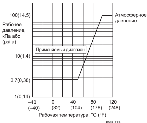
Рисунок 1. Температура процесса и рабочее давление
